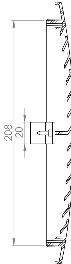
PRZEKRÓJ A-A SKALA 1 : 2
