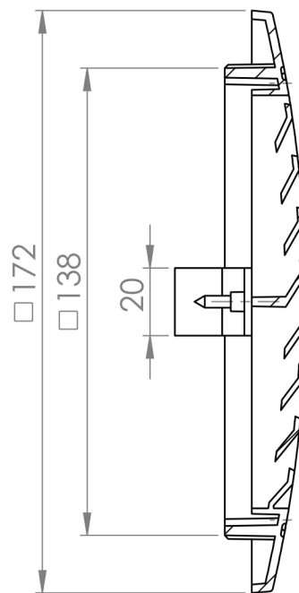
PRZEKRÓJ A-A SKALA 1 : 2
