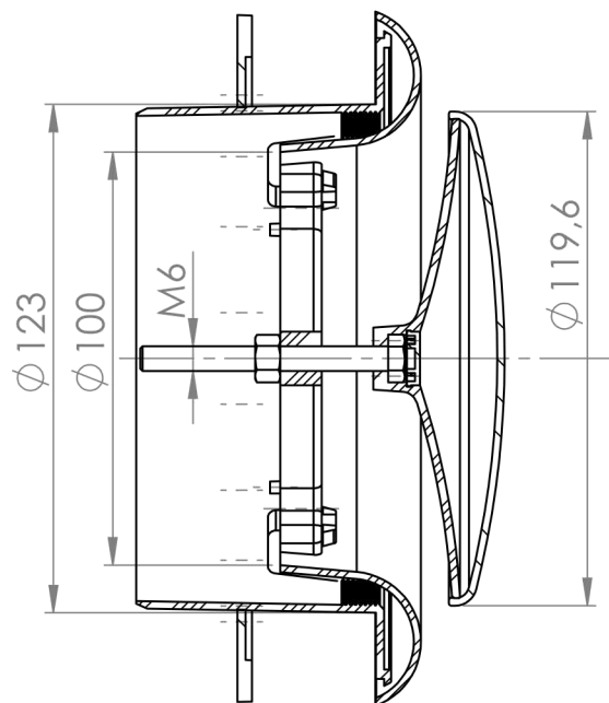
PRZEKRÓJ A-A SKALA 1 : 2
