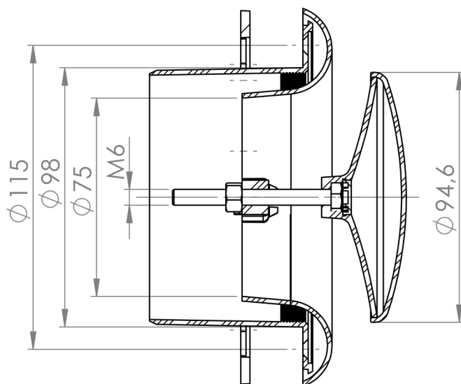
PRZEKRÓJ A-A SKALA 1 : 2
